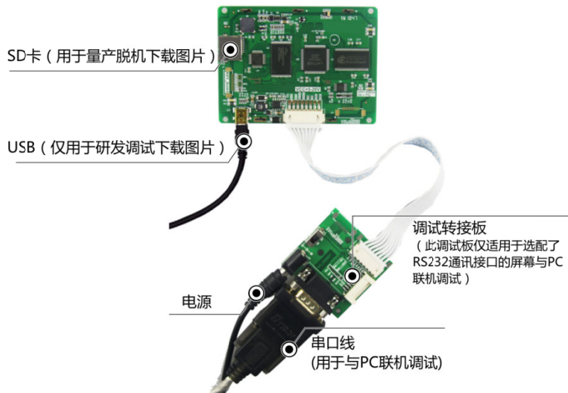
图 1-4 调试工具图
