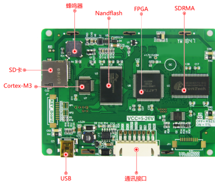
图 1-3 硬件配置图
